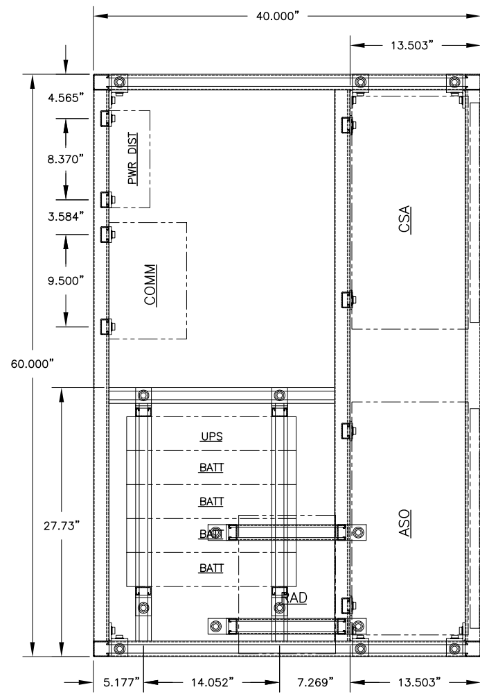
VIEW A-A
